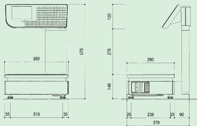
equa 3000LOOK H TESTA ALTA
